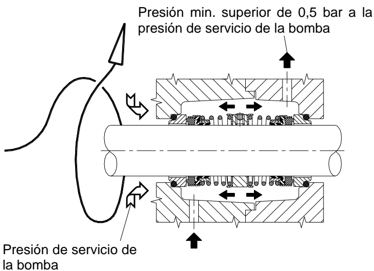
Fig. 29 Ejemplo típico de cierre mecánico DOBLE EN OPOSICIÓN auto lubricado externamente – API Plan 54
