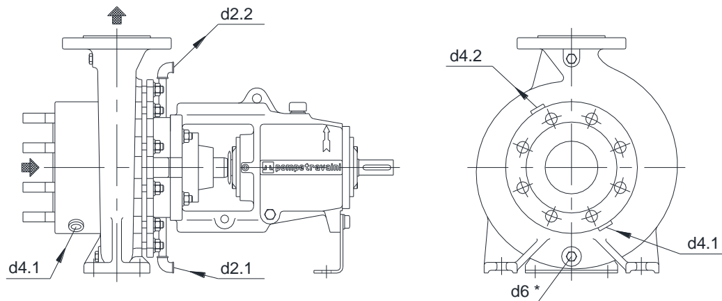
Bombas serie MC... - TC... Orificios para las versiones /T - /U2 (* = Sólo cuando está presente)
