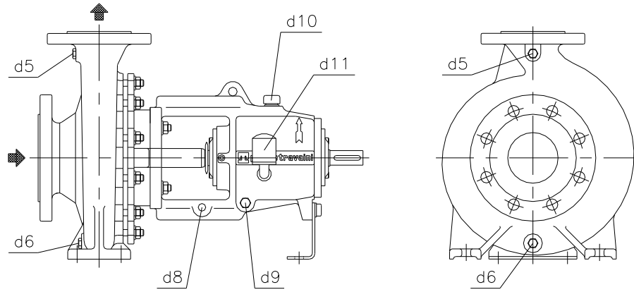
Bombas serie MC... - TC... Orificios y conexiones de serie
