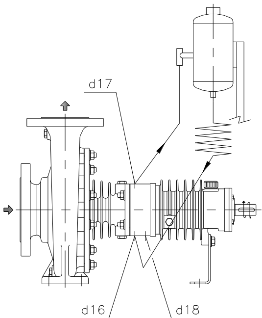
Bombas serie TCD/SP Flushing al cierre mecánico mediante Depósito
