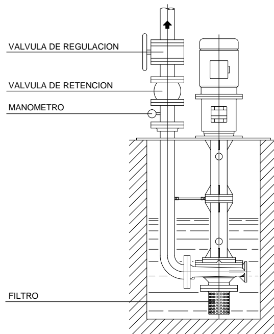
Bombas serie MC... - TC... en ejecución VERTICAL
