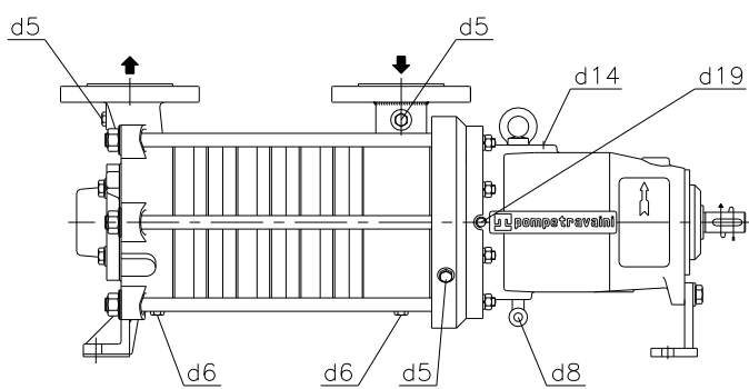
Bombas serie TBK Orificios y conexiones de serie
