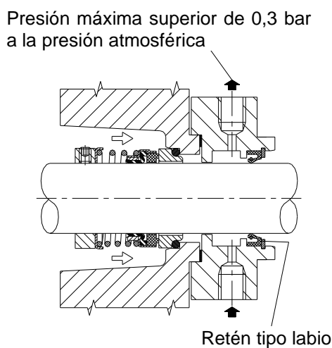
Fig. 32 Ejemplo típico de cierre mecánico SIMPLE con QUENCH – API Plan 01/62
