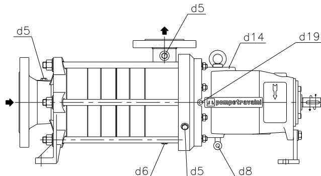
Bombas serie TBAK Orificios y conexiones de serie
